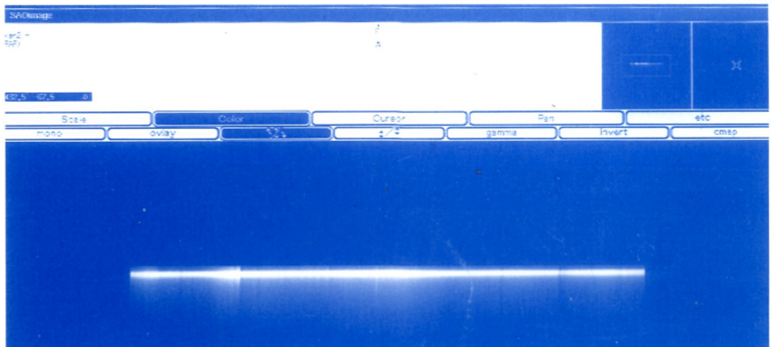
上の分光器で撮影されたハールポップ彗星のスペクトル（藤井貢氏）
